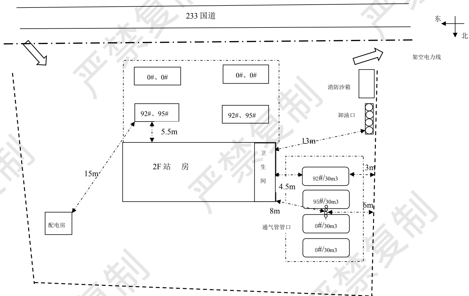
内部平面布置示意图（未标注安全间距见报告表 5-2）
