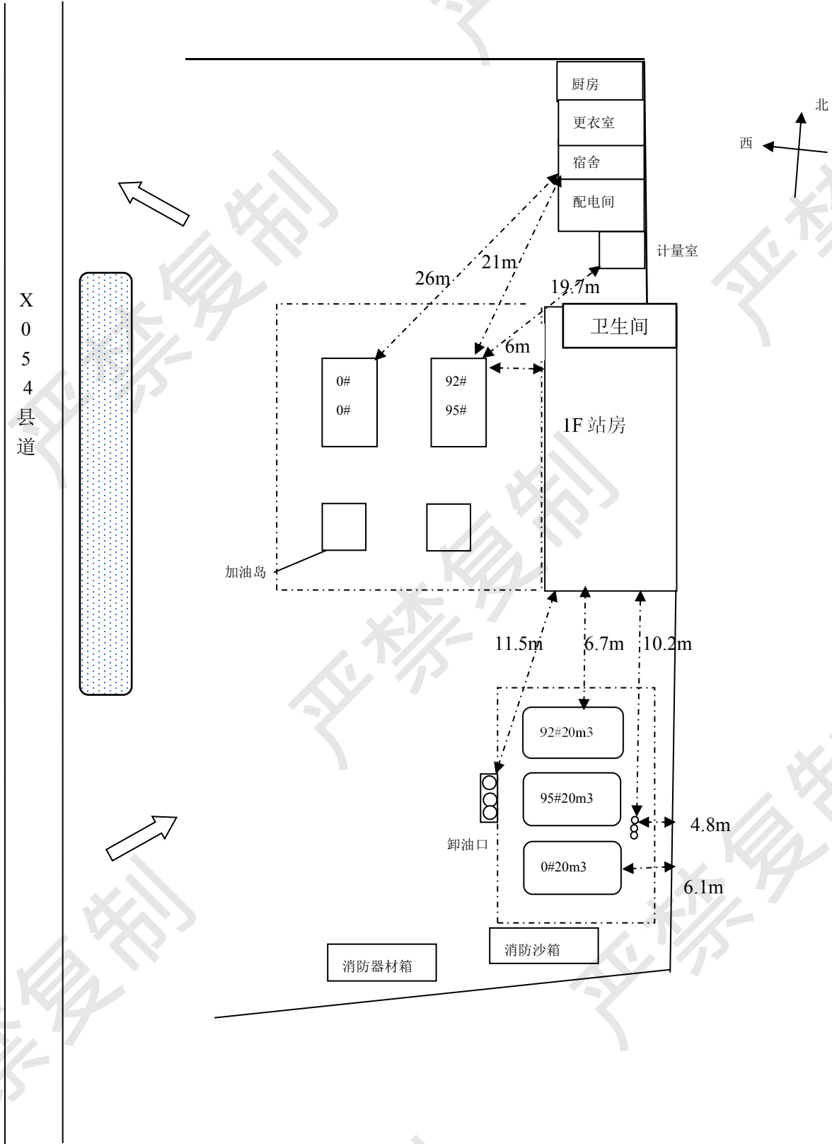
内部平面布置示意图（未标注安全间距见报告表 5-2）
