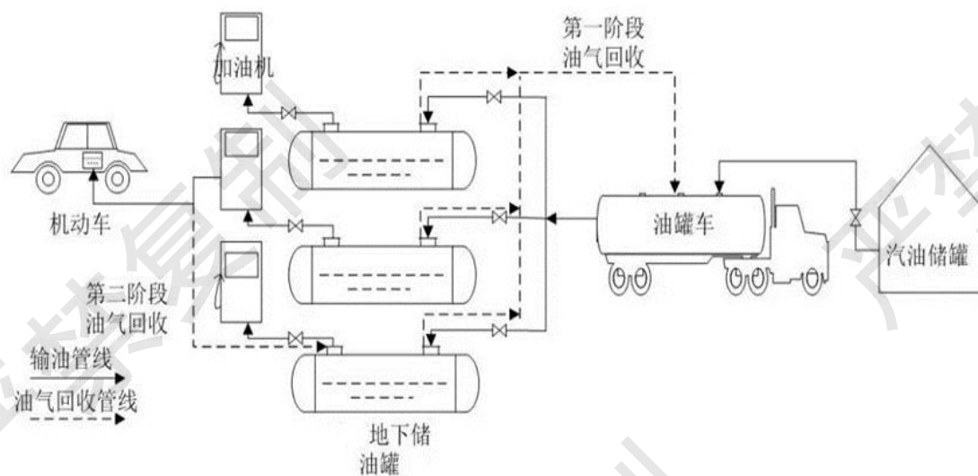
图 2-3 加油站油气回收系统示意图
