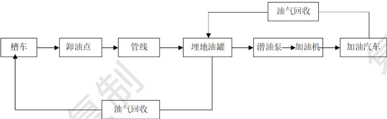
图 2-1 汽油卸油、加油流程图
