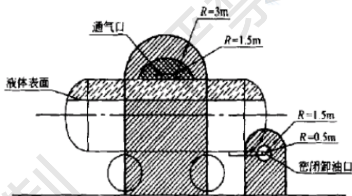
图 3-3 油罐车卸油时爆炸危险区域划分
