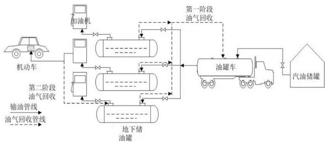
图 1-3 加油站油气回收系统示意图
