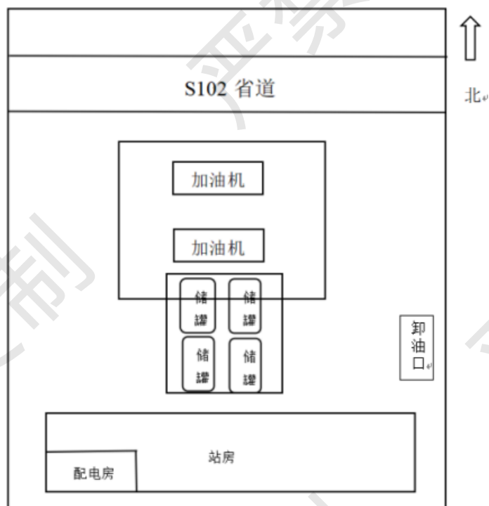
图 2-1 加油站总平面布置图
