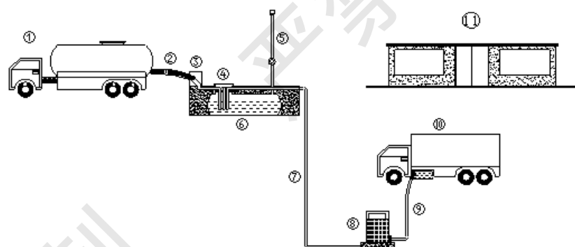
图 2-3 加油站工艺流程图
