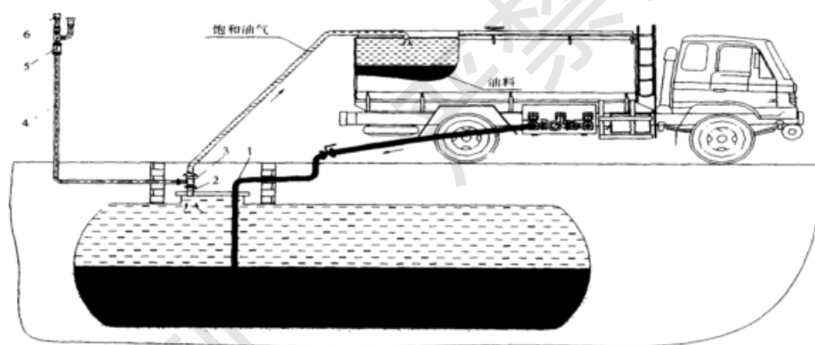
图 2-7 第一阶段油气回收系统示意图
