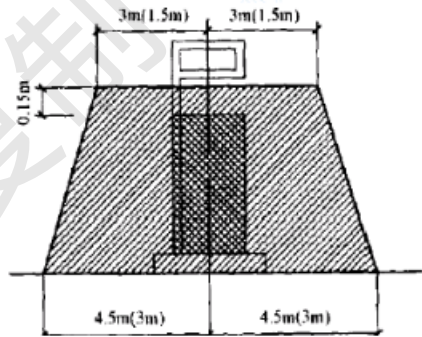
图 3-2 加油机操作危险区域划分
