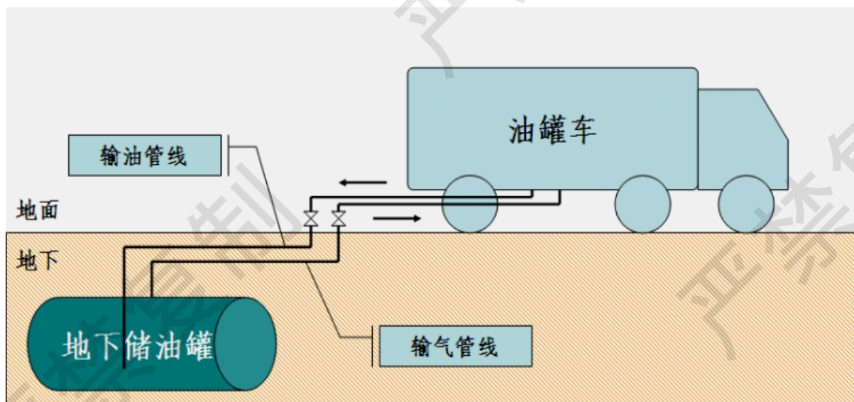
图 2-3 卸油油气回收工艺流程图
