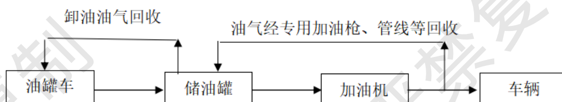
图 2-2 加油站工艺流程图
