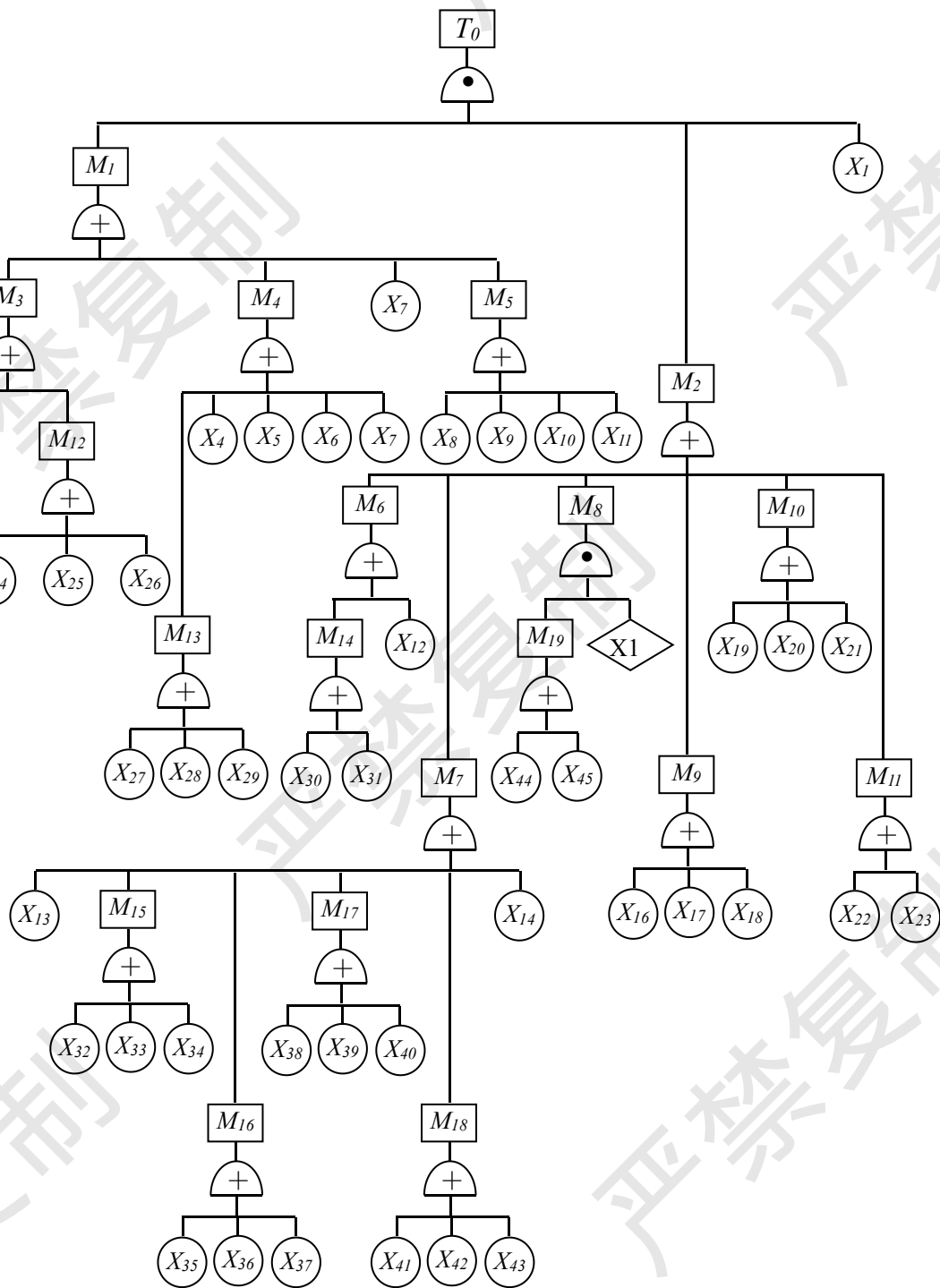
图 5-1 加油站事故树分析
