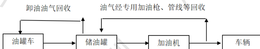
图 2-2 加油站工艺流程图
