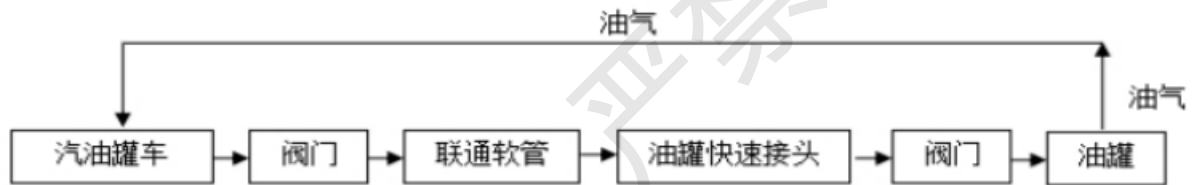
卸油工艺流程方块图
