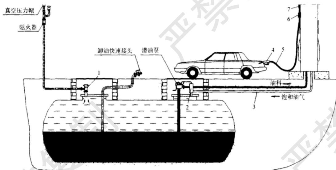
图 2-3 第二阶段油气回收系统示意图
