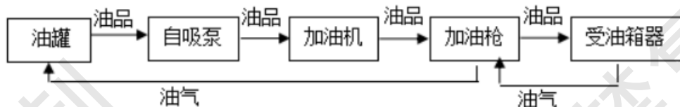
汽油加油工艺流程图
