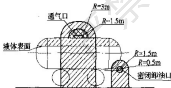
图 C.0.4 汽油的地面油罐、油罐车和密闭卸油口 爆炸危险区域划分
