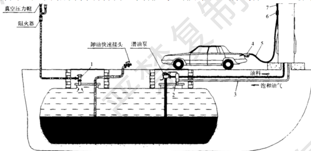
图 2-3 第二阶段油气回收系统示意图
