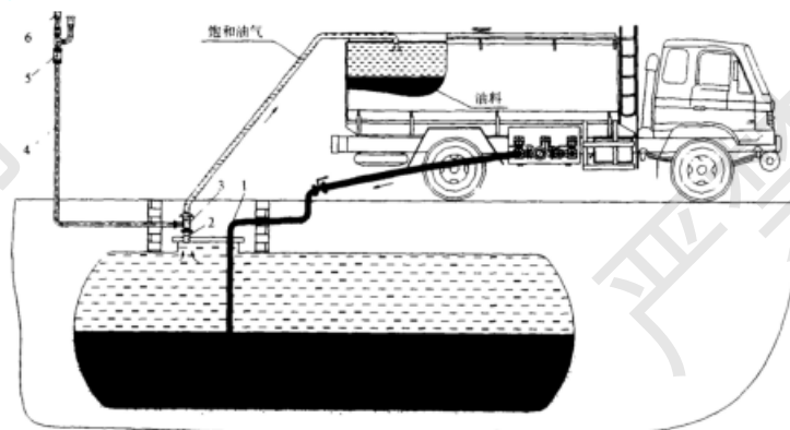
图2-2 第一阶段油气回收系统示意图
